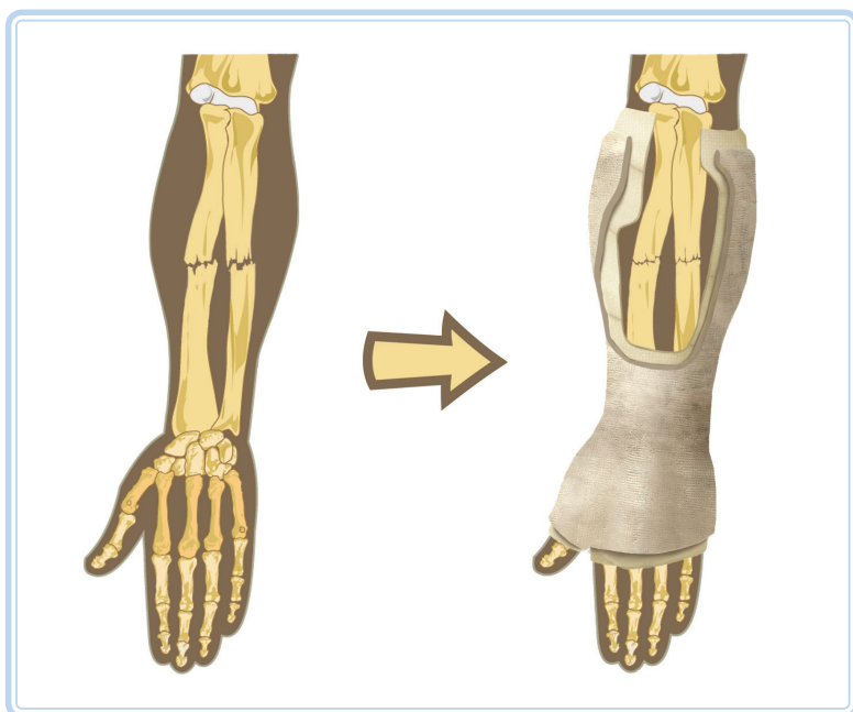
Figura 11.20: Imobilização gessada
