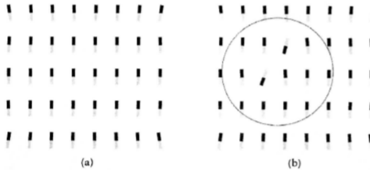
FIGURA 6-2. (a) Um arranjo de ímãs, imperfeitamente equilibrados nas beiradas. (b) Um novo arranjo, provocado pelos dois ímãs que foram desviados.
