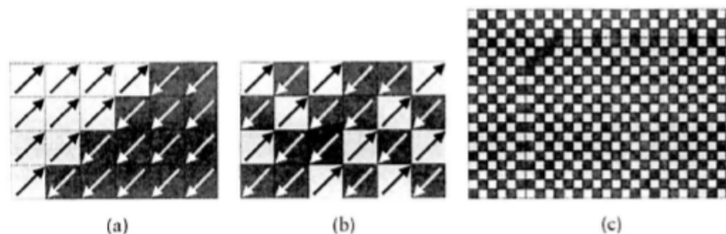
FIGURA 6-3. (a) Rotações eletrônicas em dois domínios de alinhamento comum. (b) Rotações de “antiferro” em dois domínios de alternância reversa. O limite é formado por uma dupla faixa diagonal de rotações voltadas para baixo e para a esquerda (setas brancas). (c) Mais rotações de “antiferro” em dois domínios antiferromagnéticos. O segmento diagonal do limite nesta ilustração é aquele que já foi mostrado em (b). Observe que o equilíbrio de forças difere, dependendo de sua direção.
