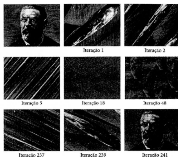
FIGURA 16-14. Transformações iteradas de um retrato de Henri Poincaré. Por volta da iteração 18, seria de presumir que nada das informações iniciais, a respeito da localização dos pixels, era recuperável. Todavia, na iteração 48, aparece uma versão com retratos superpostos e, na iteração 241, uma recorrência quase (mas não inteiramente) perfeita. Esses padrões recorrentes são conhecidos como “recorrências de Poincaré”, homenageando o homem que os descobriu.
