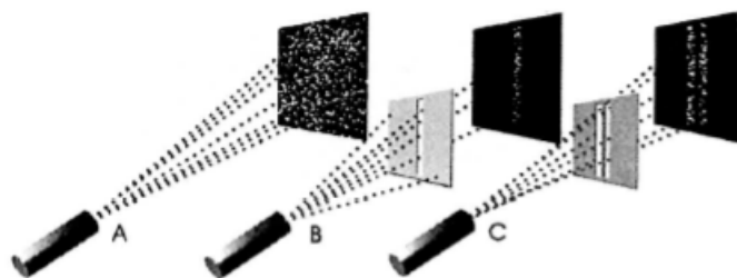
FIGURA 11-1. Chumbinhos atingindo um alvo. (A) Sem barreira. (B) Barreira de fenda única. (C) Barreira de fenda dupla.
