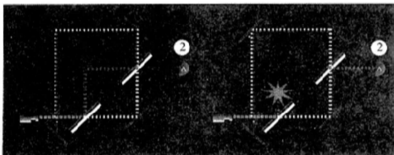
FIGURA 13-10. Um detector quântico de bombas com um único fóton (à esquerda). Não são detectadas bombas no ponto três. O fóton é retransmitido para o sistema. (À direita) Existe uma bomba no ponto três: o fóton é detectado pelo Detector nº 2 ou captado pelo disparador da bomba.
