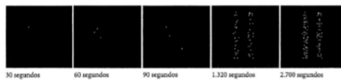
FIGURA 11-9. Espera-se que muitos elétrons individuais atinjam o espaço dentro das linhas pontilhadas que são determinadas por todas as trajetórias possíveis que cada elétron individual possa seguir através de qualquer uma das duas fendas abertas (os tempos registrados são hipotéticos).
