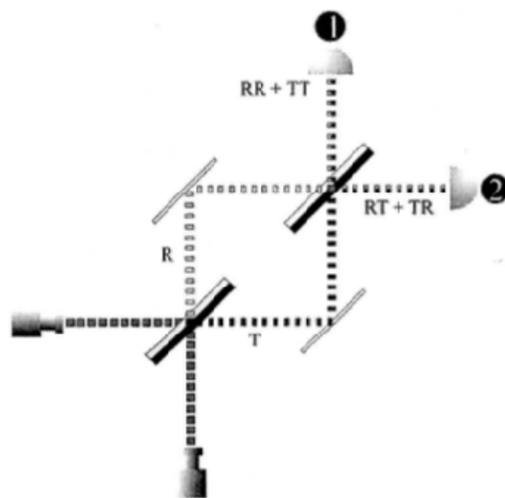
FIGURA 13-5. Um segundo separador de feixes que tanto recompina como divide os feixes previamente divididos. Para chegar ao Detector nº 1, um fóton pode ser refletido duas vezes e transmitido duas vezes (RR ou TT). Para atingir o Detector nº 2, deve ser refletido uma vez e transmitido uma vez (RT ou TR). São mostradas duas ondas de um quarto da altura inicial, que se combinam em cada detector. (Não estamos contando aqui as reflexões provenientes de qualquer um dos dois espelhos regulares.)
