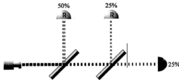
FIGURA 13-3. Realidade: depois de passar através de um separador de feixes luminosos que permite apenas a passagem de puros fótons T, um segundo separador de feixes, de algum modo, realeia os fótons T em proporções iguais de T e de R.
