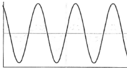
FIGURA C-1. Três ondas fasadas se combinam para formar uma única onda de amplitude maior. As três ondas são mostradas como linhas em cinza-claro colocadas umas sobre as outras, porém não somadas. A linha negra mostra as mesmas três ondas, agora somadas para formar uma única onda.
