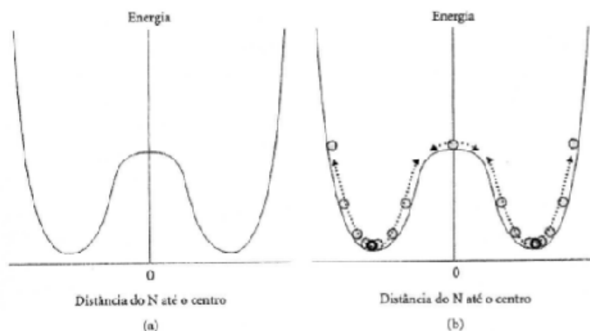
FIGURA 12-5. (a) Paisagem de energia simétrica para \text{NH}_3 . (b) O átomo de nitrogênio da amônia ocupa várias posições em ambos os lados do pico de energia.
