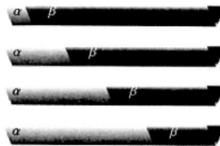
FIGURA B-2. Encrespamento conformacional viajando ao longo de um microtúbulo. Aqui, “α” representa um domínio em que o elétron móvel se encontra na subunidade “α” das proteínas das moléculas de tubulina, orientando o dipolo na direção que deve percorrer. “β” representa um domínio em que o elétron móvel se acha na subunidade “β” das proteínas da tubulina.
