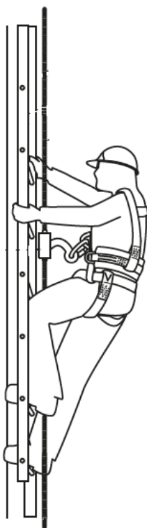
Figura 26. Exemplo de um sistema de retenção de queda baseado em uma linha de ancoragem vertical flexível instalada de forma temporária. Fonte: NBR 16489
