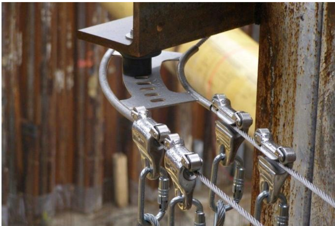
Figura 25. Exemplo de linha de vida horizontal dupla, que permite que um trabalhador passe por outro sem necessidade de se desconectar
